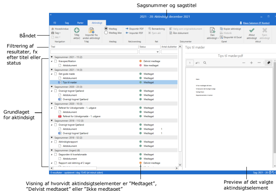
Figur 3: Fanen "Aktindsigt" i sagsvinduet
