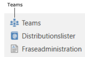
Figur 103: Menupunktet "Teams"
