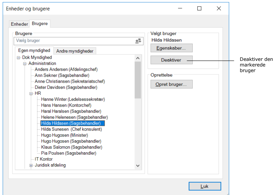
Figur 22: Deaktiver bruger
