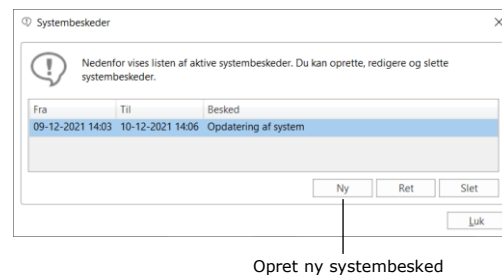
Figur 94: Dialogen "Systembeskeder"
