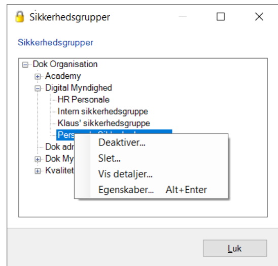
Figur 71: Deaktivér sikkerhedsgruppe
