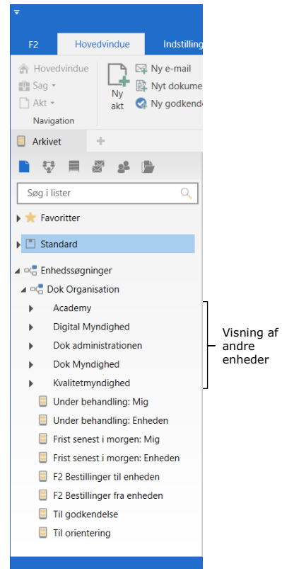
Figur 109: Enhedsoversigt
