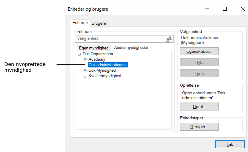
Figur 8: Nyoprettet myndighed
