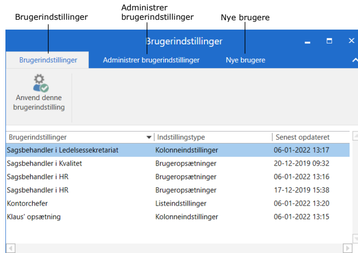
Figur 116: Dialogen "Brugerindstillinger"
