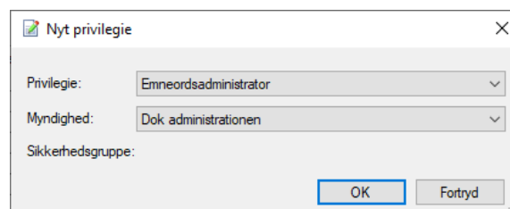
Figur 58: Privilegiet "Emneordsadministrator"
