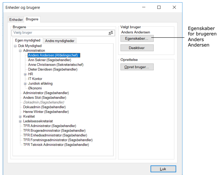
Figur 41: Udpeg bruger
