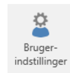
Figur 115: Menupunktet "Brugerindstillinger"
