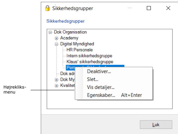
Figur 68: Dialogen "Sikkerhedsgrupper"
