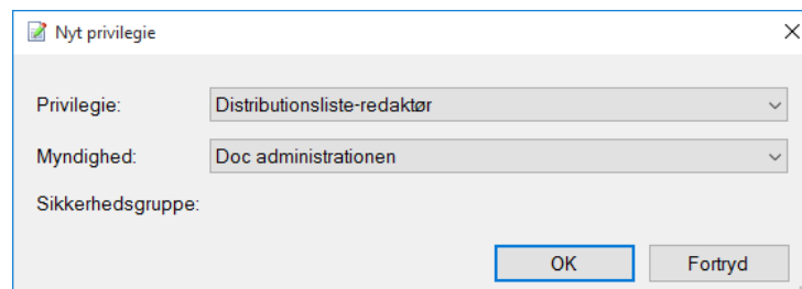
Figur 57: Privilegiet "Distributionsliste-redaktør"
