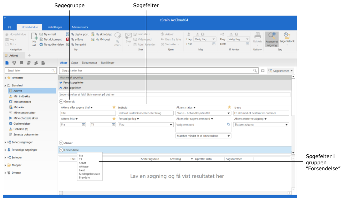
Figur 106: Avanceret søgning
