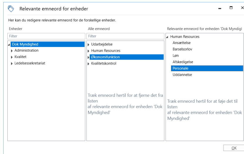
Figur 92: Udvælg emneord
