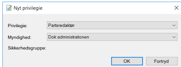
Figur 60: Privilegiet "Partsredaktør"
