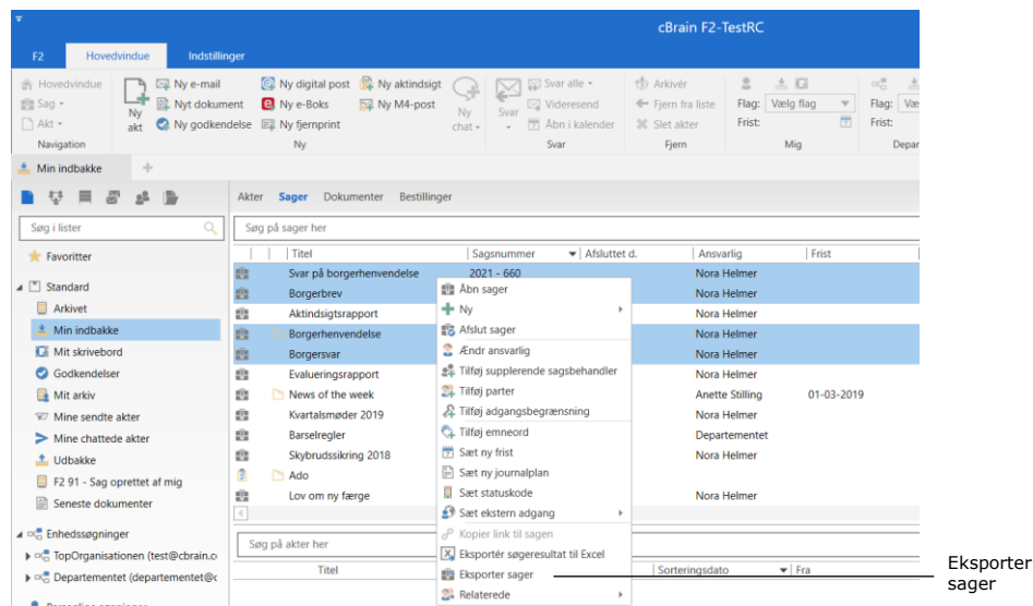
Figur 2: Eksporter sager
