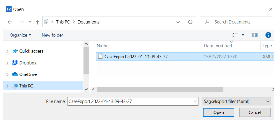
Figur 9: Find eksporfiler
