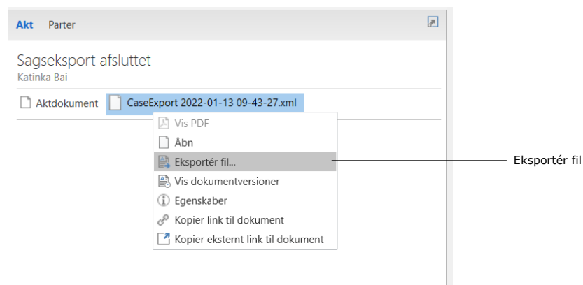
Figur 6: Eksportér eksportfil
