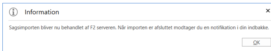
Figur 11: Informationsboks - Import
