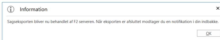
Figur 4: Informationsboks - Eksport
